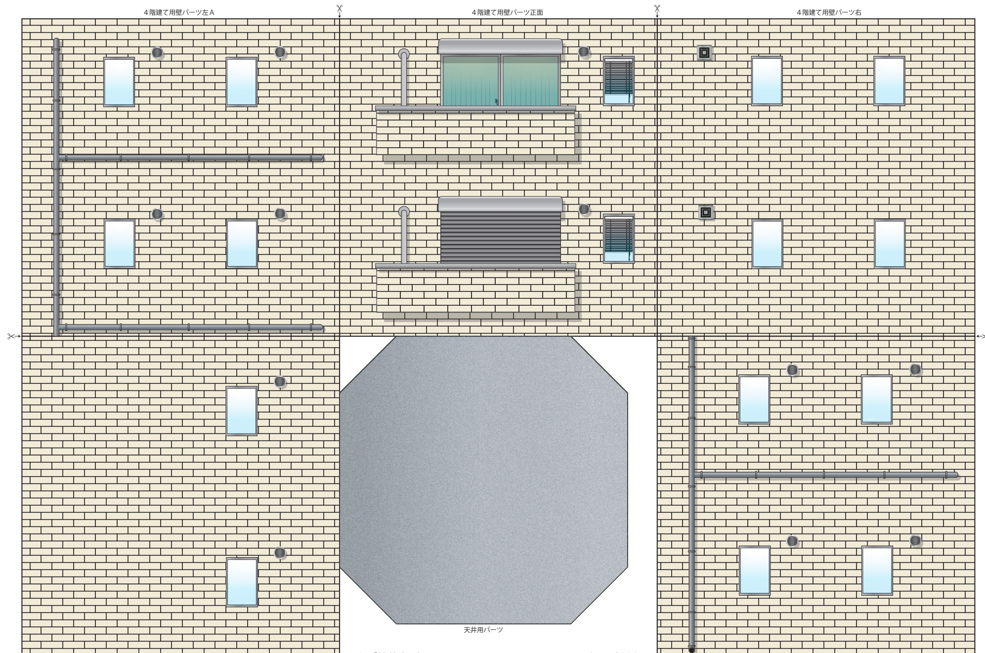
4階建て用壁パーツ左B ※このパーツを2階建て部分の左側に使用してください
